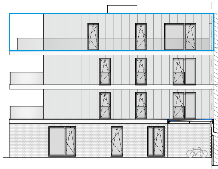
Achtergevel
